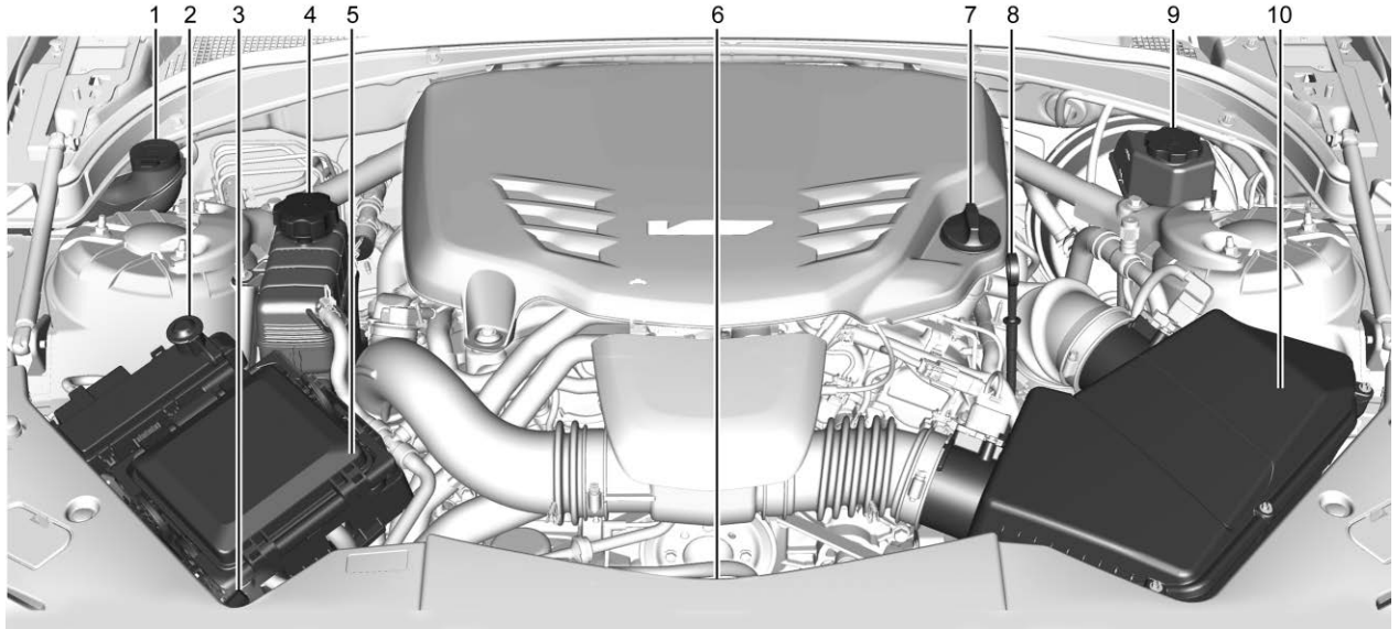
محرك تربييني مزجود V6 سعة ٣,٦ لتر (LF4)
